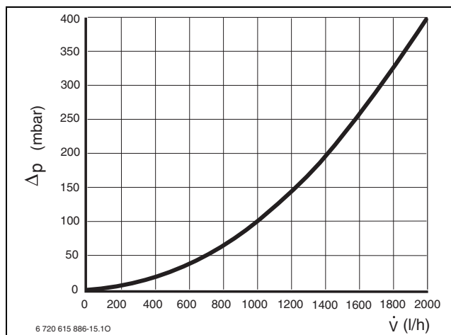
Рис 6 Потеря давления в котле BWC 42
