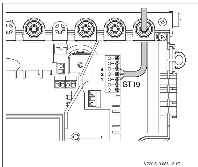
Рис 20 Подключение 24 В регулятора
