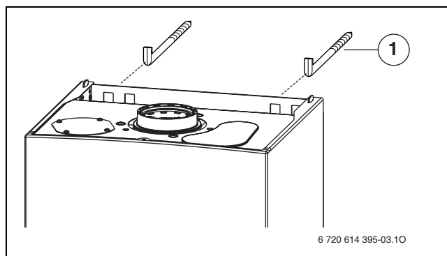
Рис 8 Подвешивание прибора
