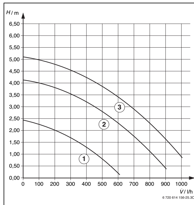
Рис 36 Характеристики насоса (без монтажной соединительной плиты)
