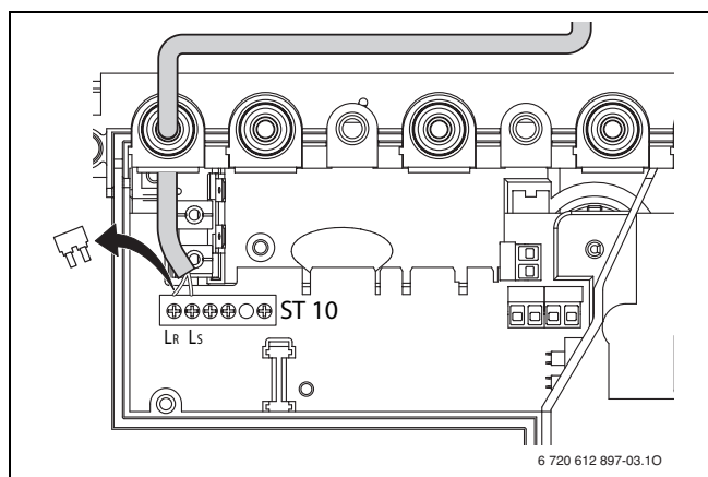
Рис 19 Подключение (230 В AC, снять перемычку между L S и L R )
