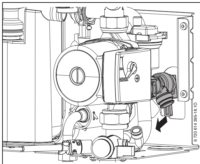
Рис 59 Предохранительный клапан (система отопления)
