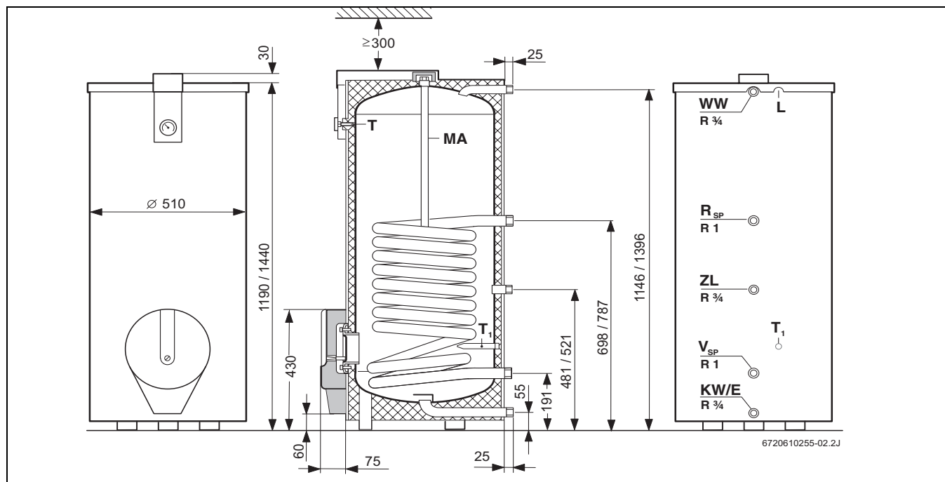
Рис 3 Размеры после косой черты относятся к следующему большому исполнению бойлера.
