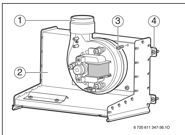
Рис 45 Вентиляторный блок
