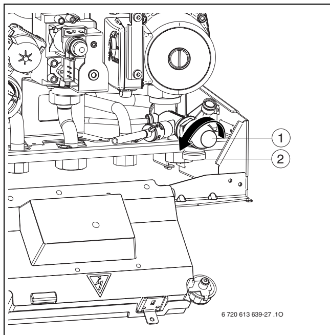
Рис 48 Предохранительный клапан
