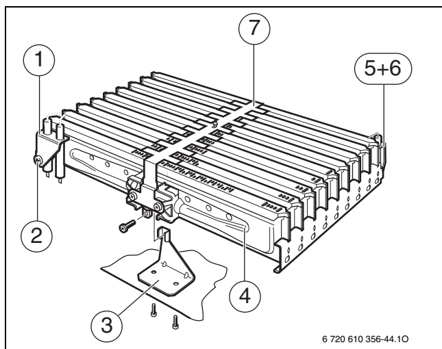
Рис 42 Узел горелки
