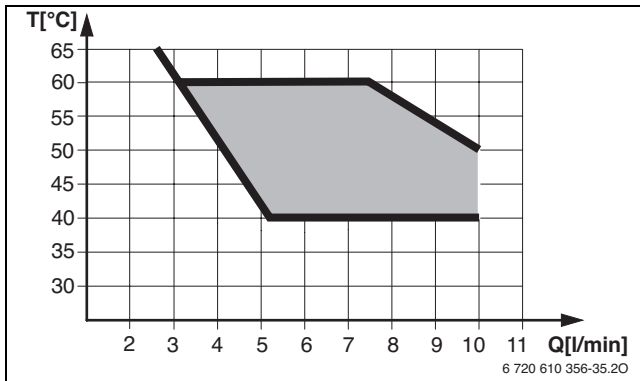
Рис 26 Диаграмма при температуре холодной воды на входе +15 °C
