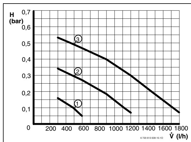
Рис. 32 Характеристики насоса
