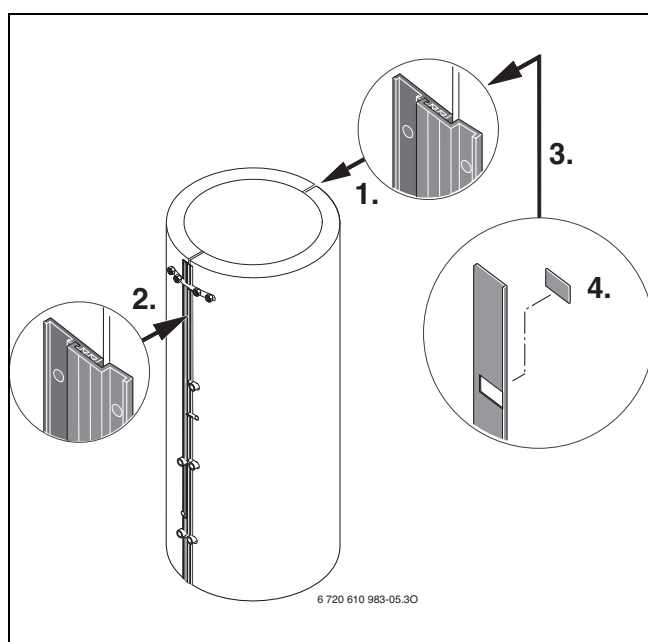
Рис 6 Замыкание соединительных планок
