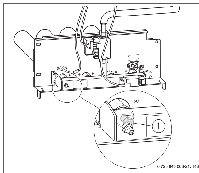
Рис. 24 Проверка форсунок
