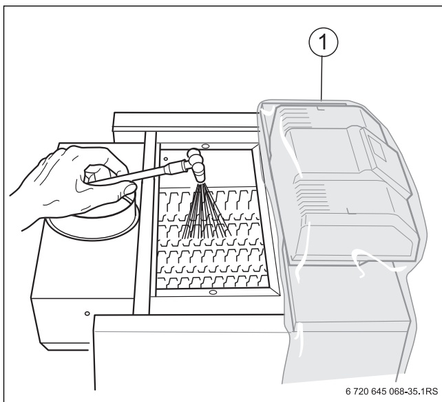
Рис. 43 Влажная чистка котла
