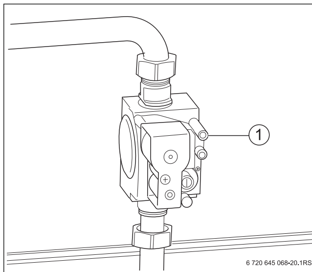
Рис. 27 Измерение подаваемого давления газа
