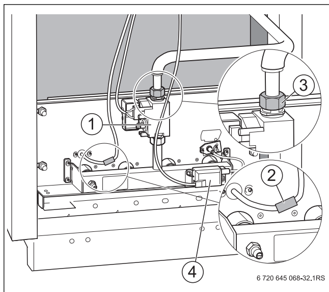
Рис. 40 Демонтаж горелки
