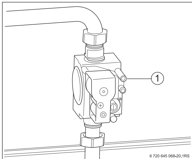
Рис. 37 Проверка внутренней герметичности
