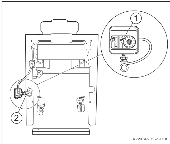
Рис. 7 Подключение газа
