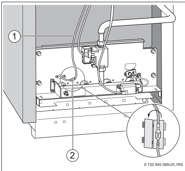
Рис. 29 Удаление защиты от касания
