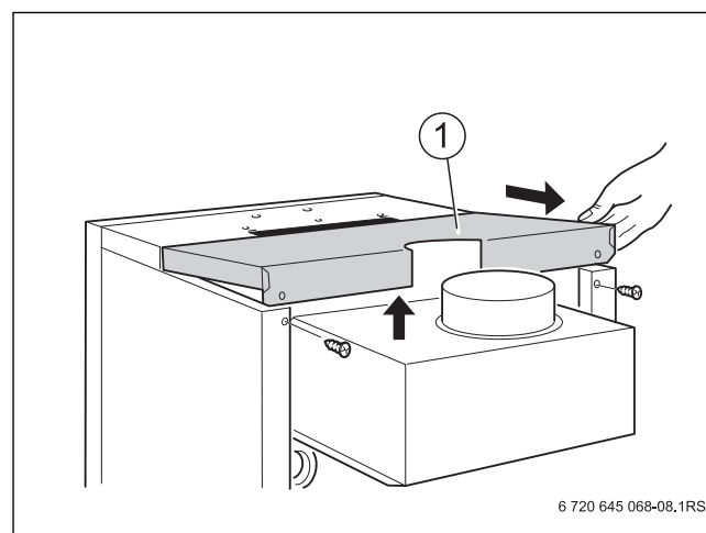
Рис. 12 Снятие задней крышки котла
