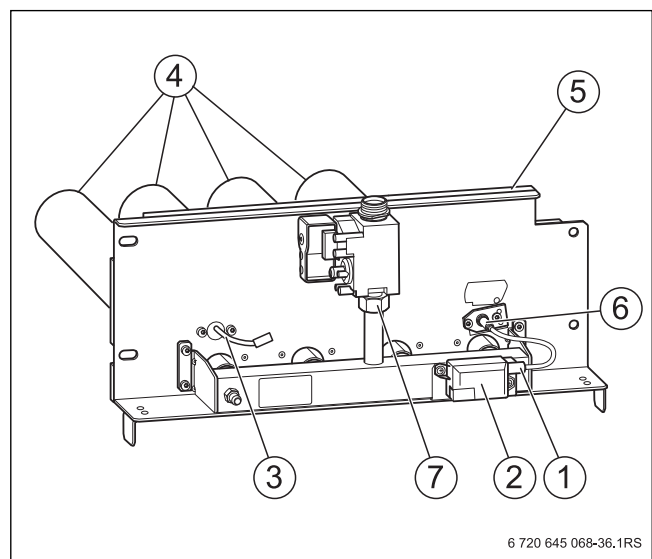
Рис. 44 Чистка горелки
