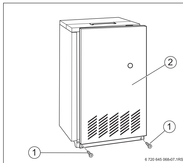
Рис. 11 Демонтаж передней стенки котла
