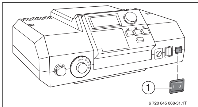
Рис. 35 Выключение отопительной установки
