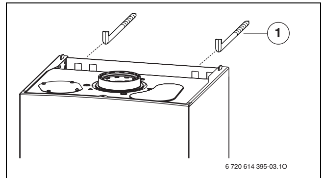
Рис 8 Подвешивание прибора
