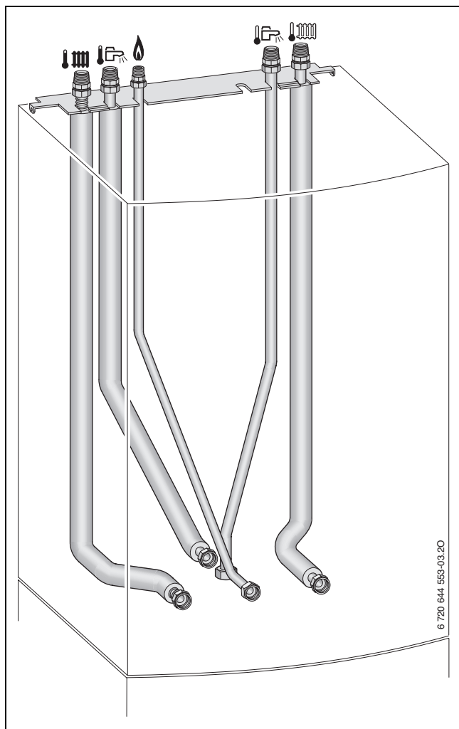
Рис 10 Пример: вертикальные подключения № 1523
