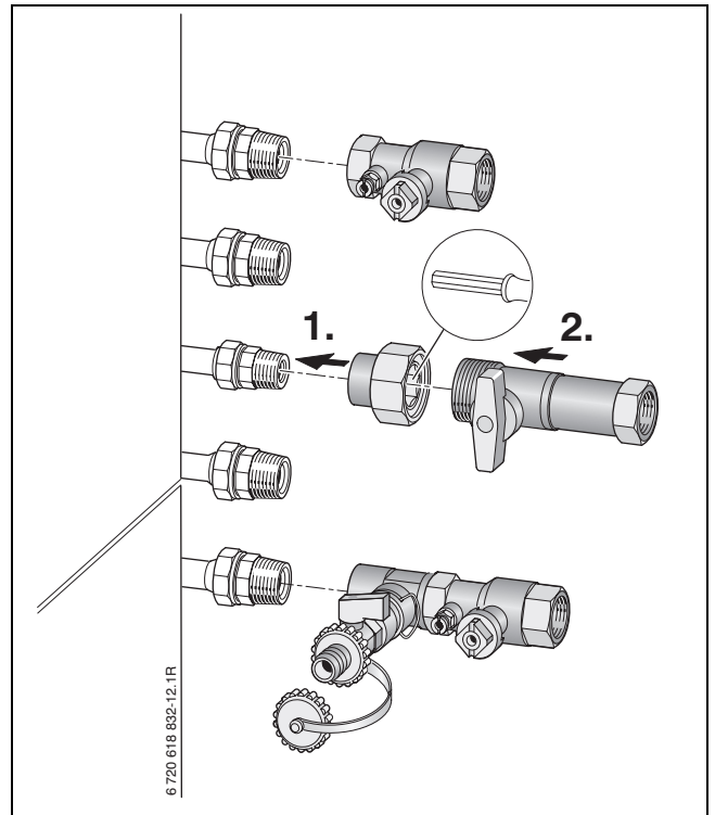
Рис 13 Монтаж сервисных кранов № 862 на примере подключений справа № 1521
