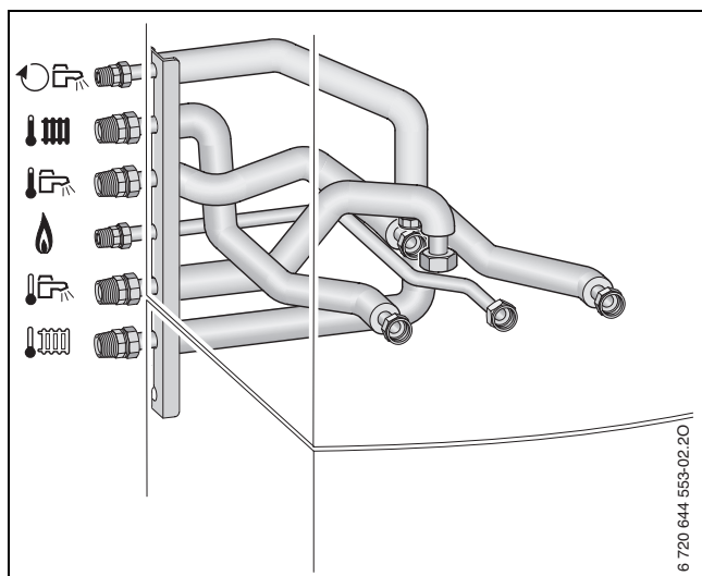
Рис 9 Пример: подключения слева № 1519
