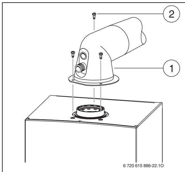
Рис 27 Монтаж системы отвода продуктов сгорания
