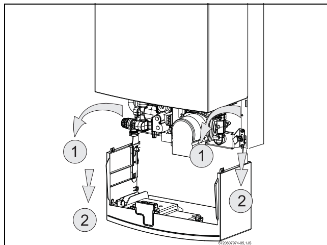
Рис. 34 Сервисное положение для доступа к системам водо- и электроснабжения
