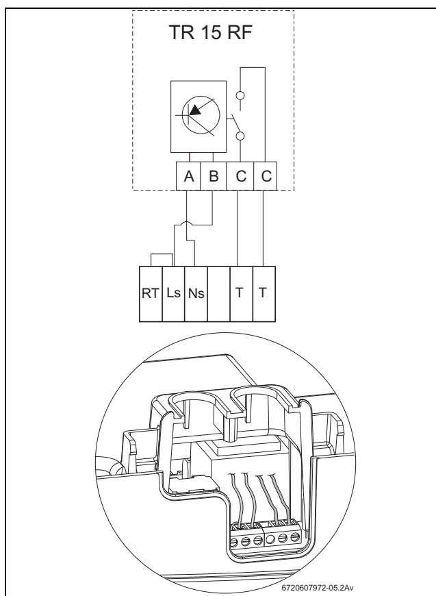
Рис. 21 TR 15 RF
