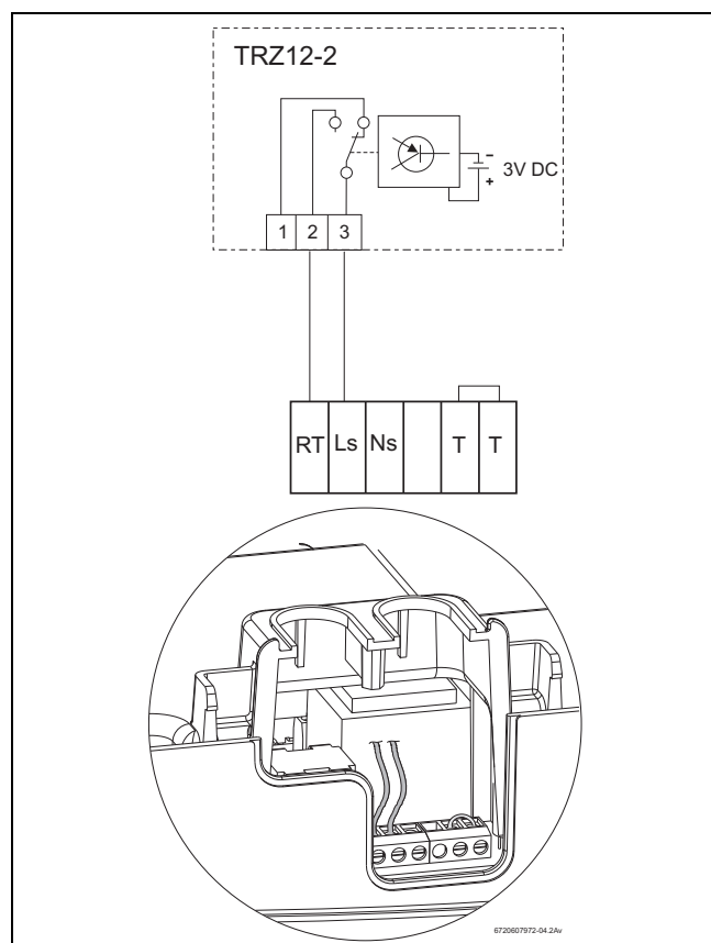
Рис. 20 TRZ 12-2
