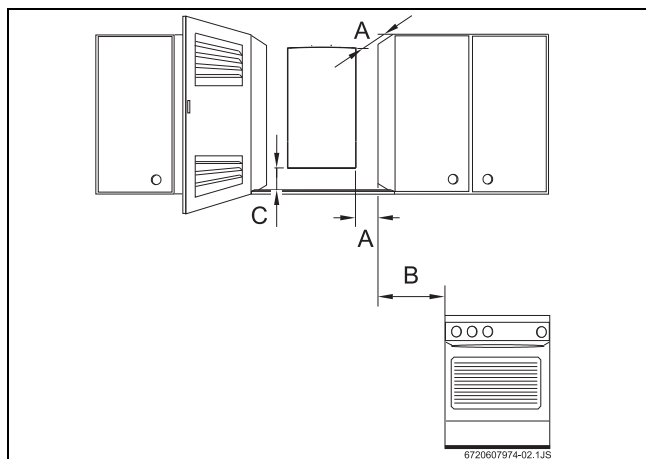
Рис. 7 Минимальные расстояния
