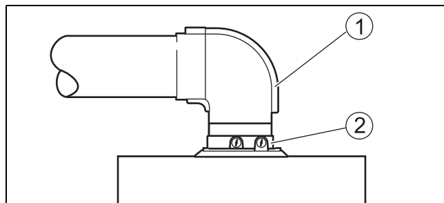
Рис. 13 Фиксация отводной коленчатой трубы при помощи зажимной клеммы
