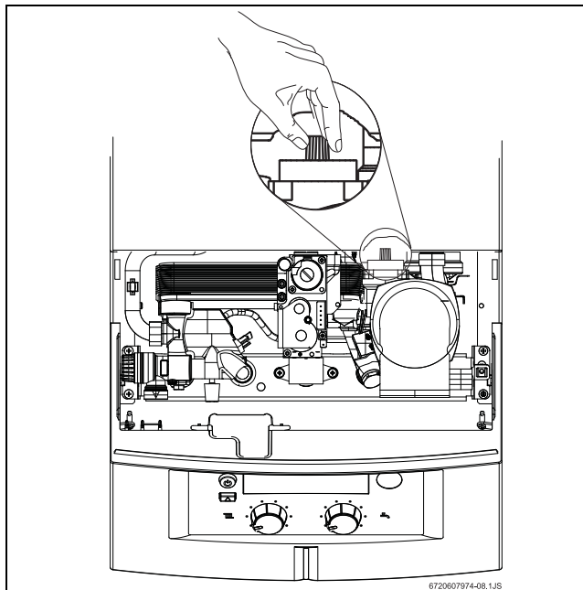
Рис. 17 Воздухоотводчик
