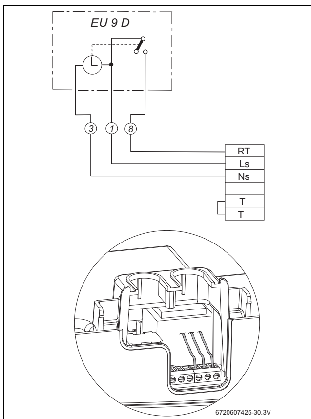
Рис. 22 EU 9 D
