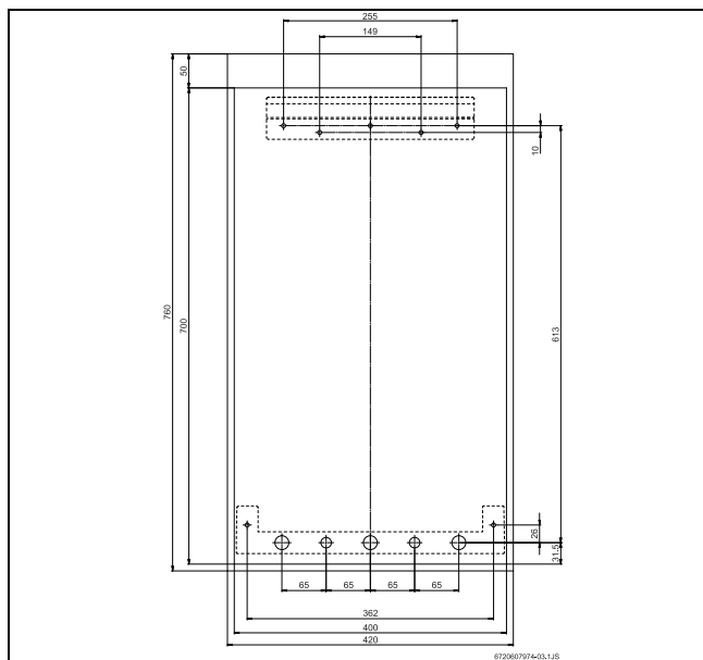
Рис. 8 Комплект для настенного монтажа
