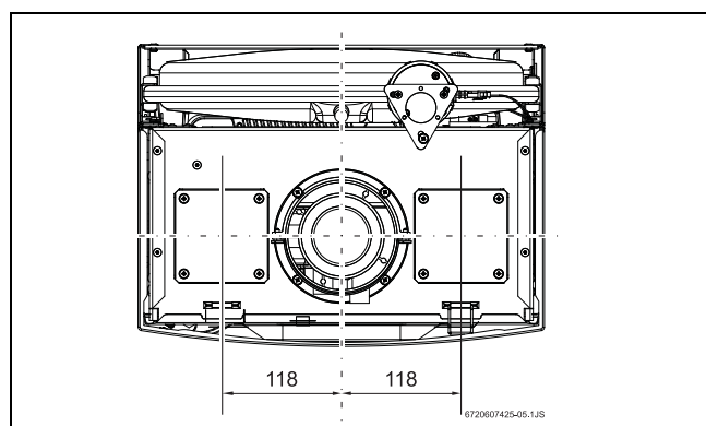
Рис. 2 Вид сверху
