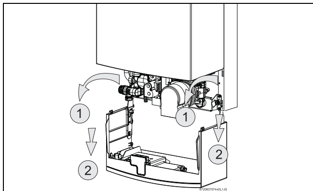
Рис. 10 Сервисное положение для доступа к системам водо- и электроснабжения
