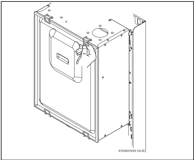
Рис. 31 Защитная панель
