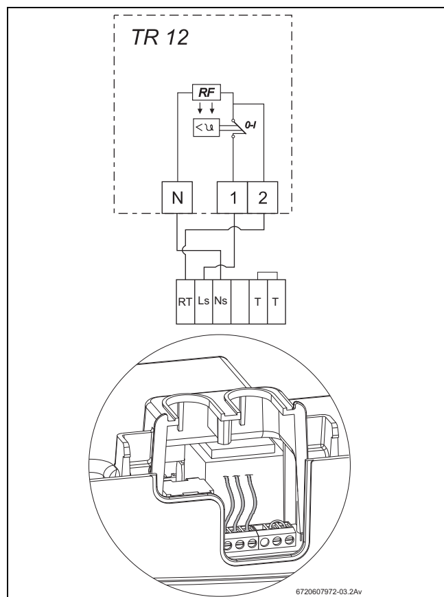
Рис. 19 TR 12
