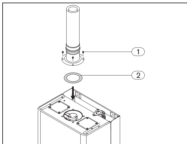
Рис. 14 Монтаж дроссельной шайбы
