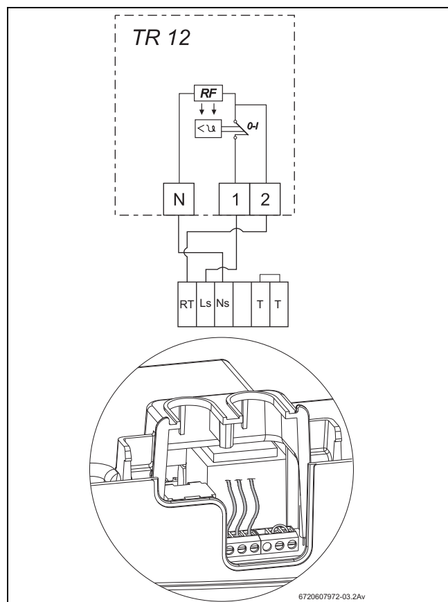
Рис. 16 TR 12
