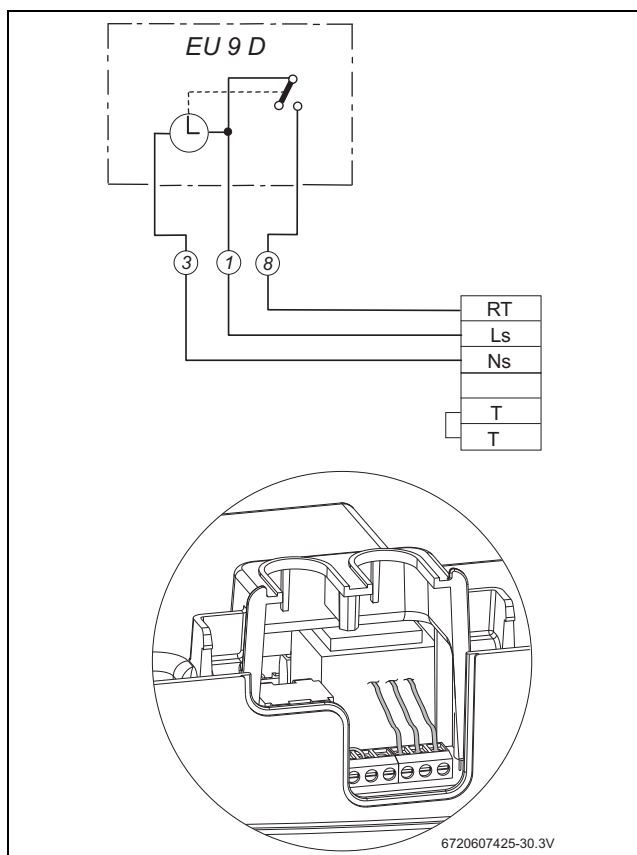
Рис. 19 EU 9 D
