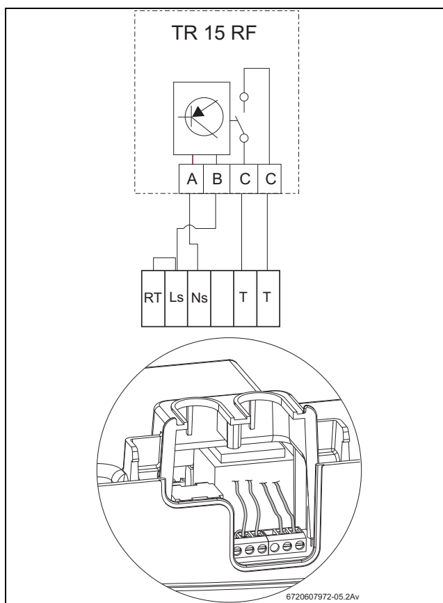
Рис. 18 TR 15 RF
