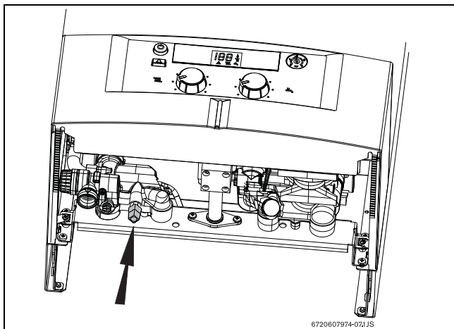
Рис. 13 Кран подпитки
