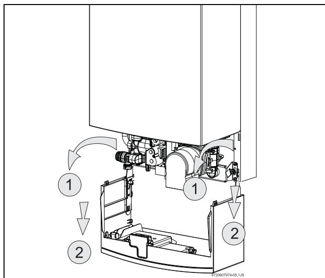
Рис. 31 Сервисное положение для доступа к системам водо- и электроснабжения
