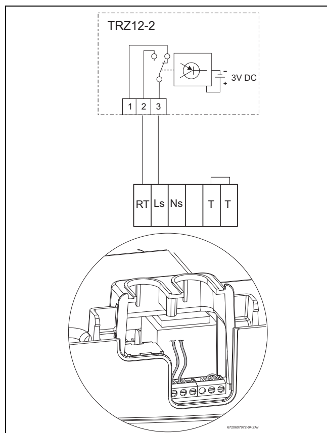
Рис. 17 TRZ 12-2
