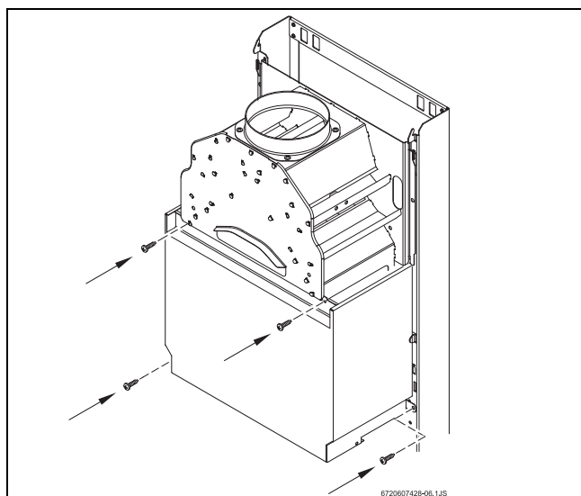
Рис. 28 Защитная панель
