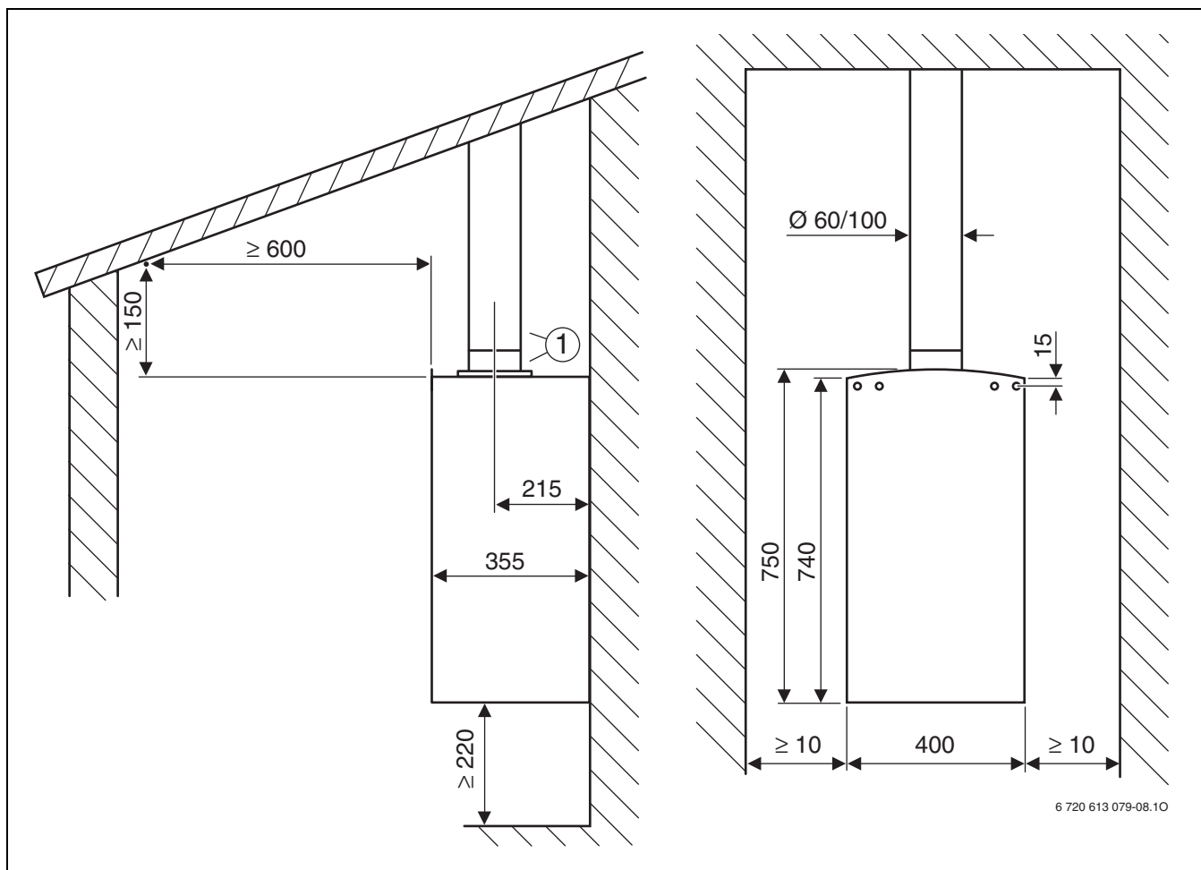
Рис 6 Наклонная крыша
