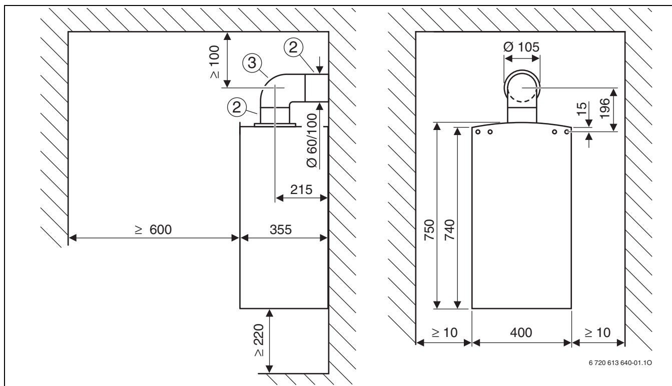
Рис 1 Отвод дымовых газов по C 12
