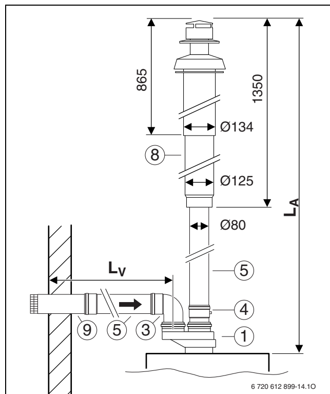
Рис 16 Отвод дымовых газов по C 52
