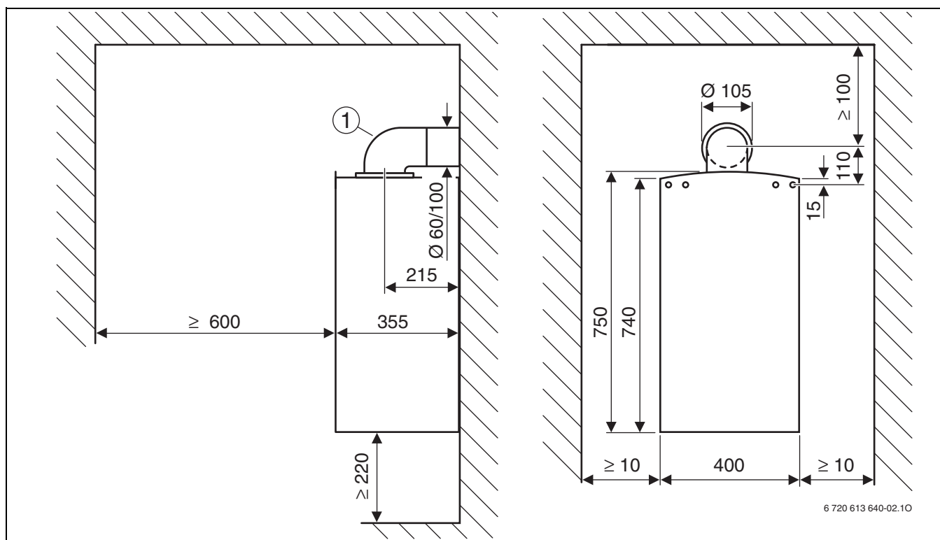
Рис 2 Отвод дымовых газов по C 12
