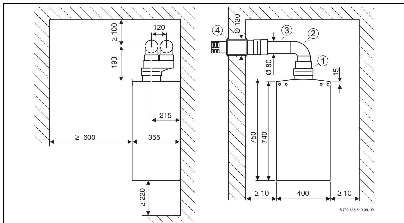
Рис 9 Отвод дымовых газов по C 12
