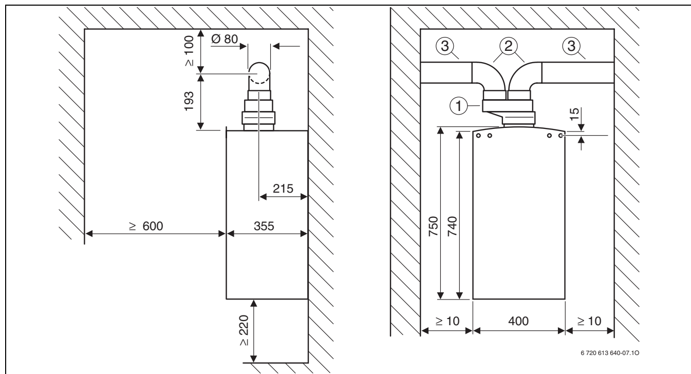
Рис 10 Отвод дымовых газов по C 42 , или C 82
