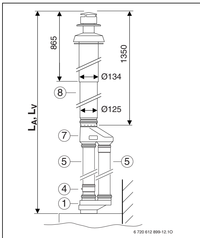
Рис 15 Отвод дымовых газов по C 32
