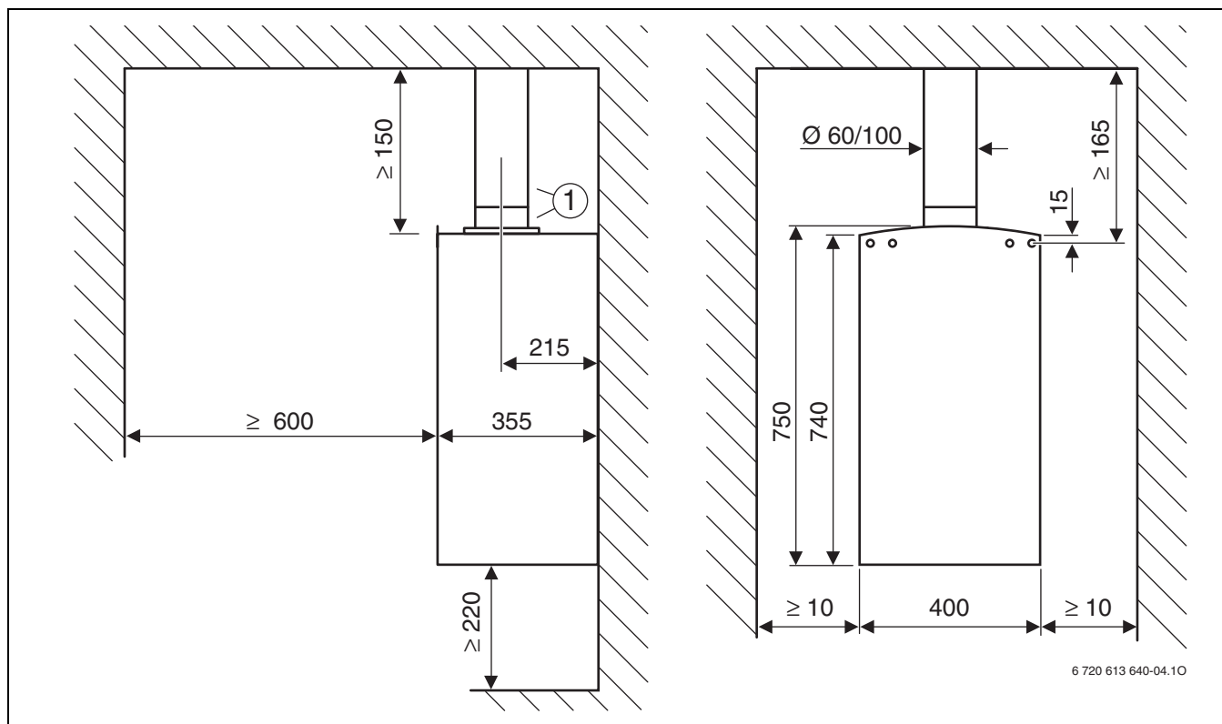
Рис 5 Плоская крыша
