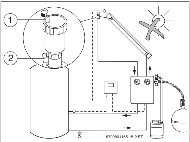
Рис. 39 Закреть запорный винт воздухоотделителя и шаровой кран
