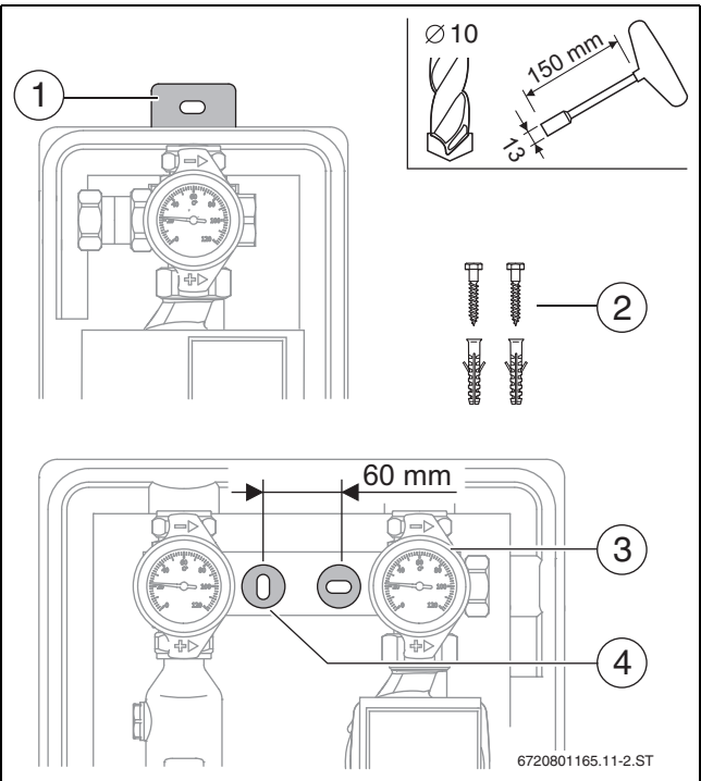
Рис. 14 Монтаж станции
