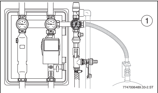
Рис. 38 Контроль стрелки манометра
