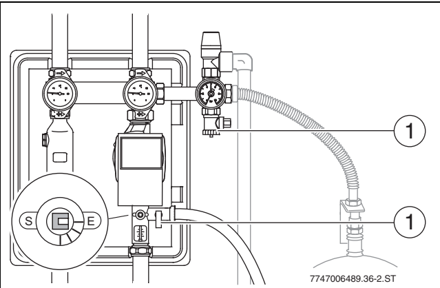
Рис. 37 Заполнение через кран для наполнения и слива
