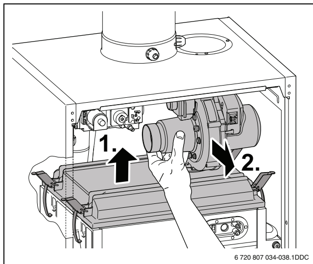
Рис. 54 Удаление газозводного блока с крышкой горелки
