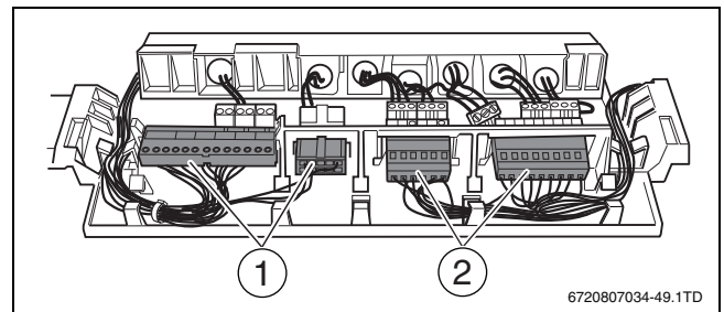
Рис. 27 Клеммные колодки
