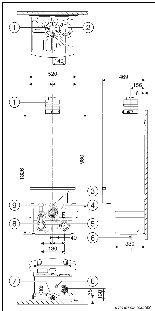
Рис. 3 Размеры [мм]
