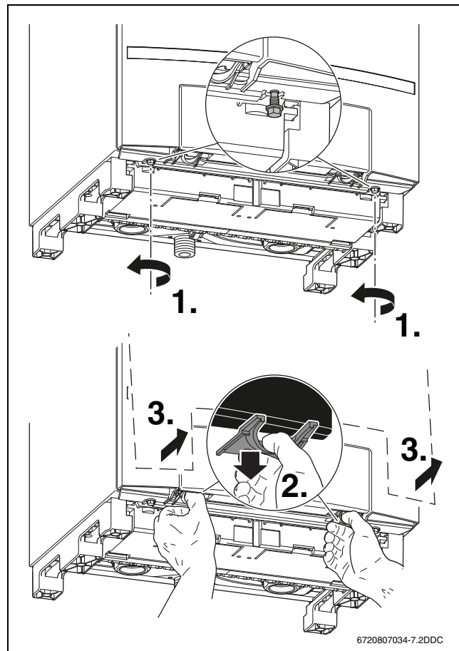
Рис. 2 Снятие облицовки
