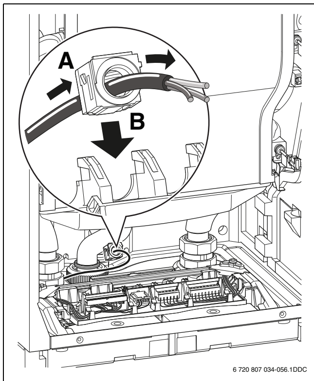
Рис. 28 Проводка провода
