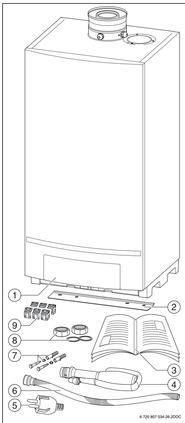
Рис. 1 Комплект поставки
