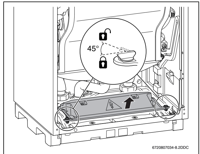
Рис. 26 Снятие крышки
