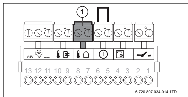
Рис. 33 Подключение датчика наружной температуры
