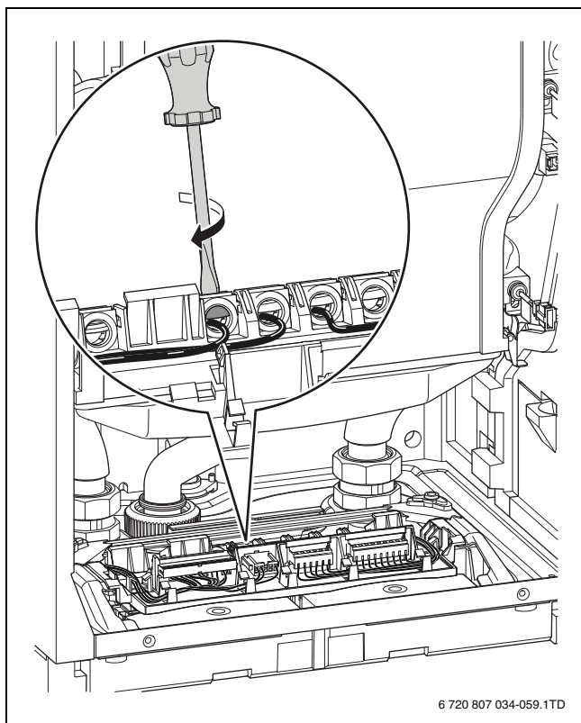
Рис. 29 Затягивание винта
