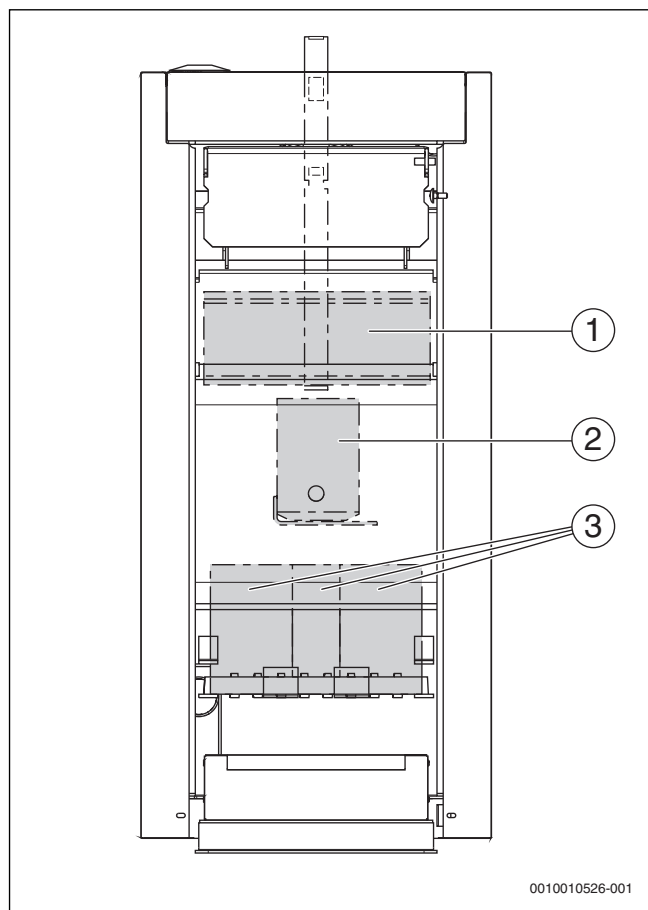
Рис. 21 Положение камней в топке (вид спереди)
