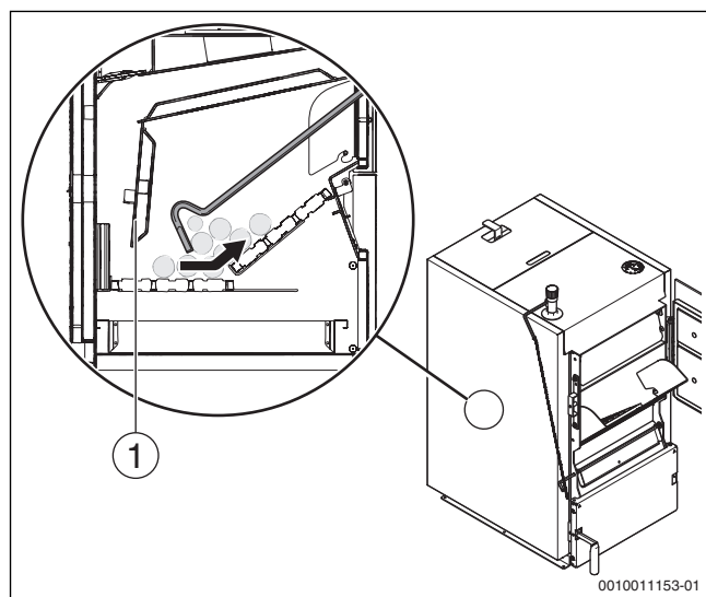
Рис. 39 Ворошите угли и очищайте пространство под пластиной
