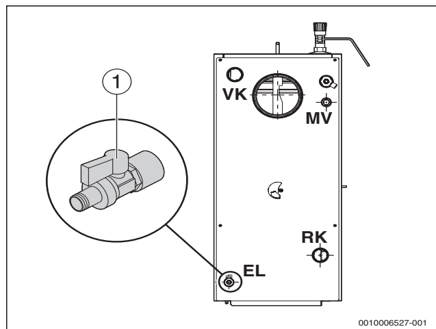
Рис. 15 Гидравлические подключения
