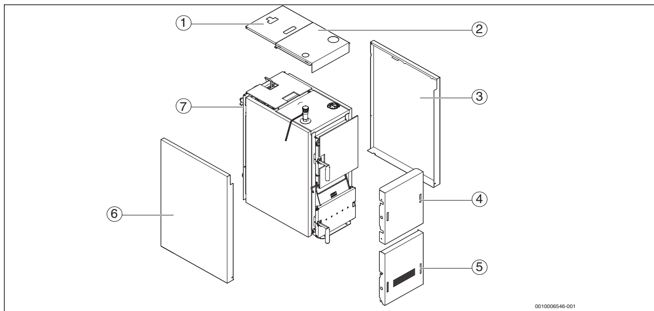
Рис. 6 Элементы облицовки котла
