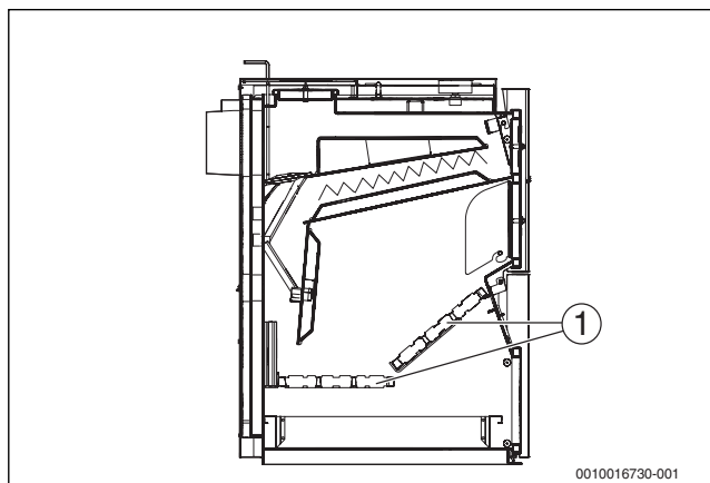
Рис. 22 Положение решёток
