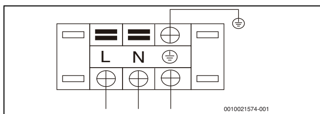
Рис. 30 Входное питание
