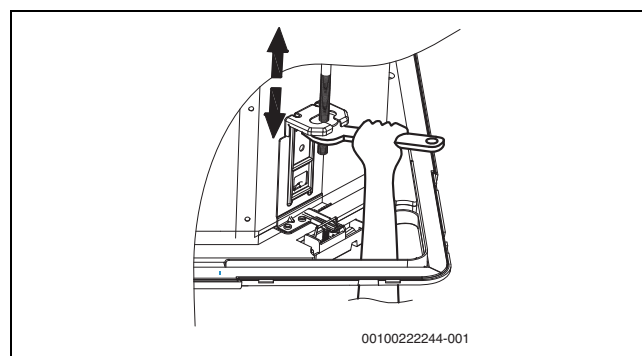
Рис. 23 Регулировка высоты внутреннего блока
