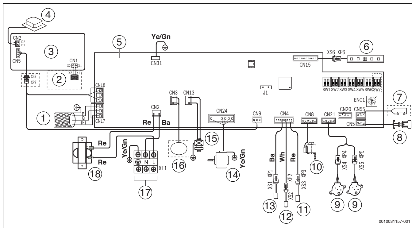
Рис. 58 Электропроводка, прототип 90–140
