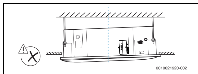
Рис. 22 Зазоров быть не должно
