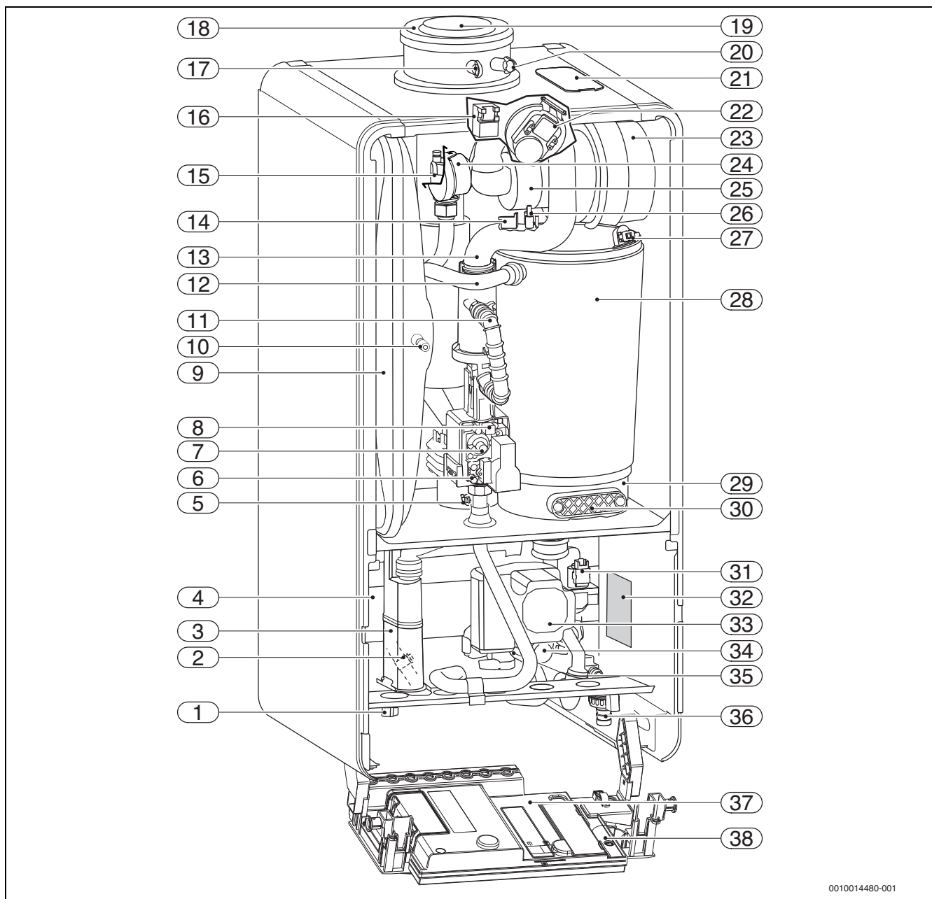
Рис. 3 Маҳсулот ҳақида умумий маълумот
