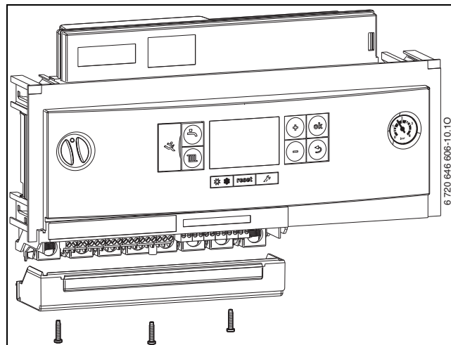
Расм 29 Қопқоқни ечиб олинг
