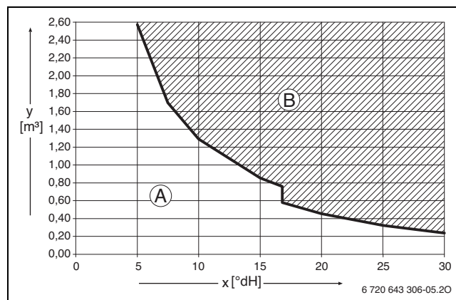
Rasm 19 Техника жиҳозлари учун қўшимча сув ва қўшимча сувга бўлган талаблар °dH < 50 кВт
