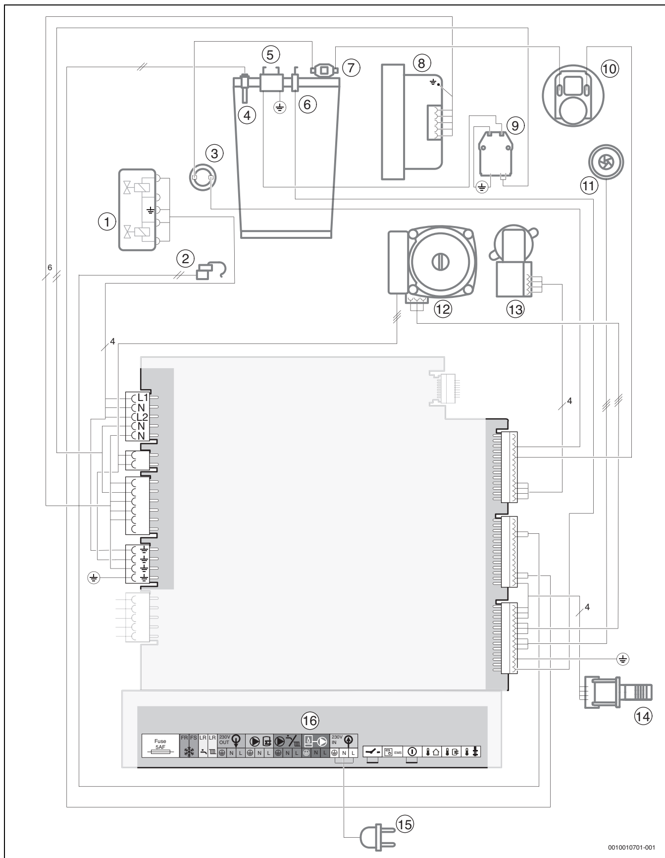
Расм 79 Электр симлари
