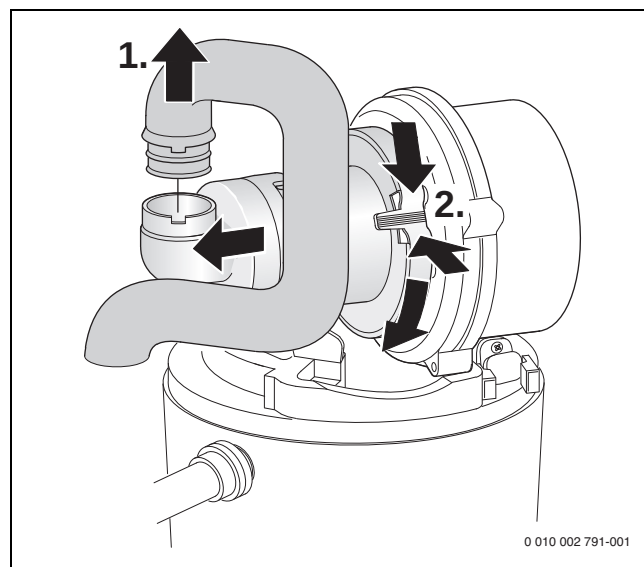
Рasm 51 Тушириш коллектори ва аралаштириш қурилмасини олиб ташланг
