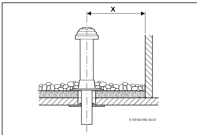
Рasm 5 Текис том учун масофа ўлчамлари
