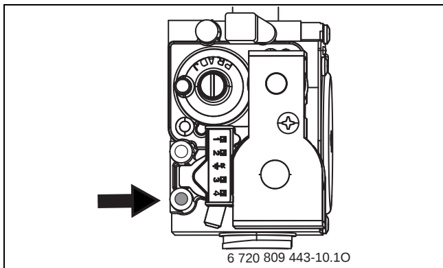
Rasm 47 Газ уланишининг босими ўлчаш мосламаси
