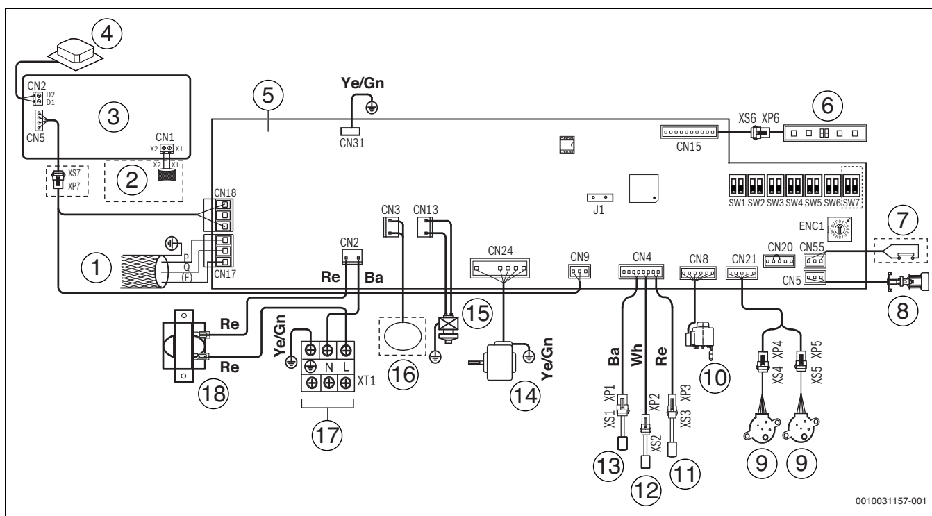
Рис. 58 Электропроводка, прототип 56–140
