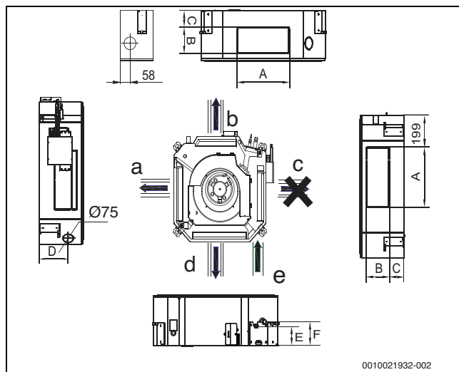
Рис. 26 Принципиальная схема монтажных размеров воздухопроводов
