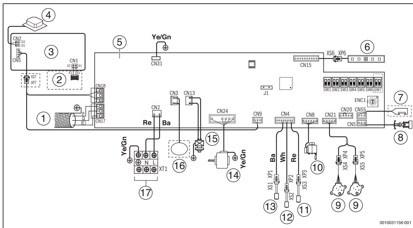
Рис. 57 Электропроводка, прототип 28-45
