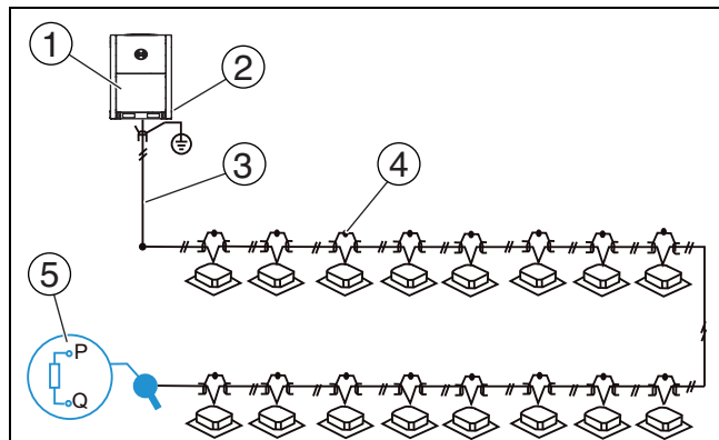
Рис. 43 Коммуникационная проводка внутренних и наружного блоков (PQE)
