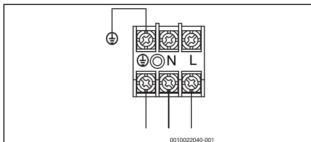
Рис. 39 Входное питание
